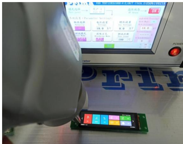
图 4-2 ESD 测试图
