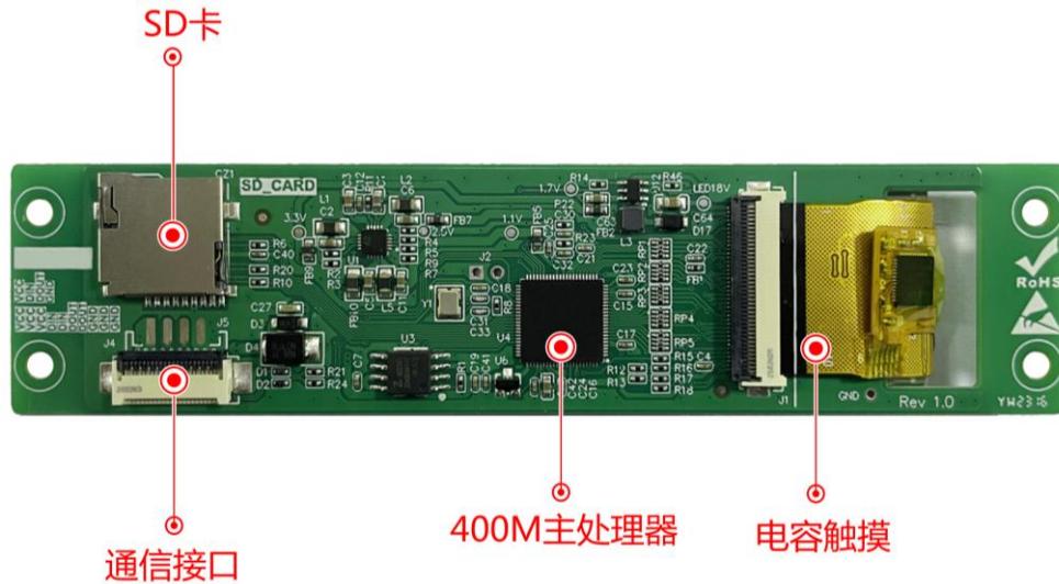
图 1-3 硬件配置图
