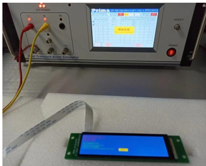
图 4-3 EFT 测试图
